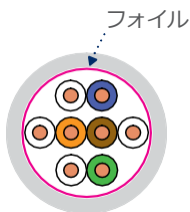
F / UTP フォイル ツイストペア
