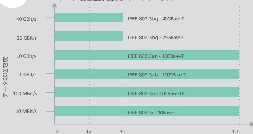
データ転送速度と長さ (4ペアケーブル)
