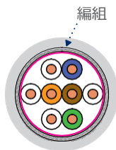
SF / UTP 編組+フォイル ツイストペア
